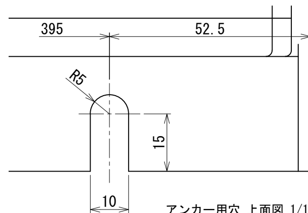
アンカー用穴 上面図 1/1
