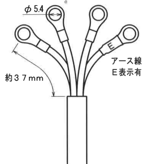
200V用電源コード 1.25sq 4芯 機械外長4m
